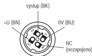
vnitřní pohled na konektor (varianta "C")
