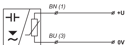
zapojení snímače s výstupem typu NAMUR (provedení "Xi", "XiM", "XiT")
