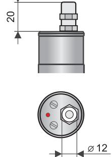
provedení "D" s kab. vývodkou
