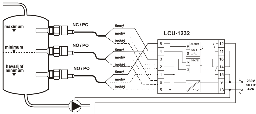
b) Regulace odčerpáváním s funkcí ALARM detekující havarijní minimum Zapojení se snímači s výstupem NPN nebo PNP (např. DLS-27N, CPS-24N)
