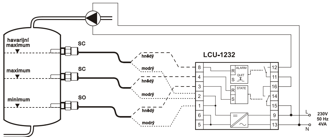
c) Regulace dočerpáváním s funkcí ALARM detekující havarijní maximum Zapojení se snímači s výstupem SO, SC (např. GPLS-25N, CLS-18)
