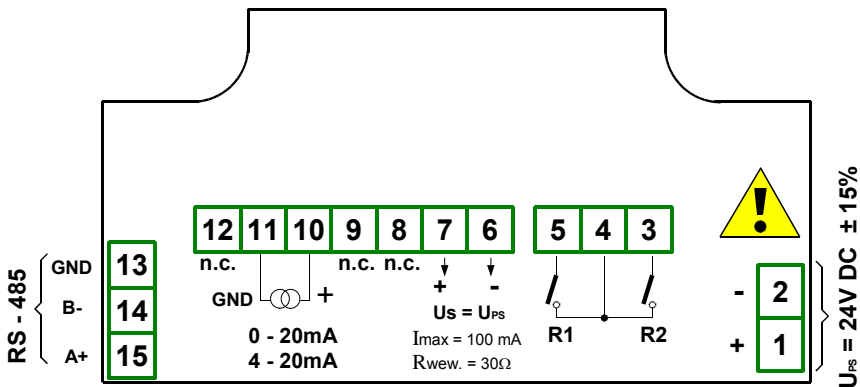
Obrázek 4.4. Zapojení svorek (verze 24V DC)
