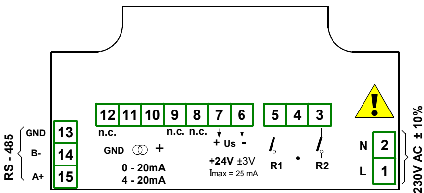
Obrázek 4.2. Zapojení svorek (verze 230V AC)
