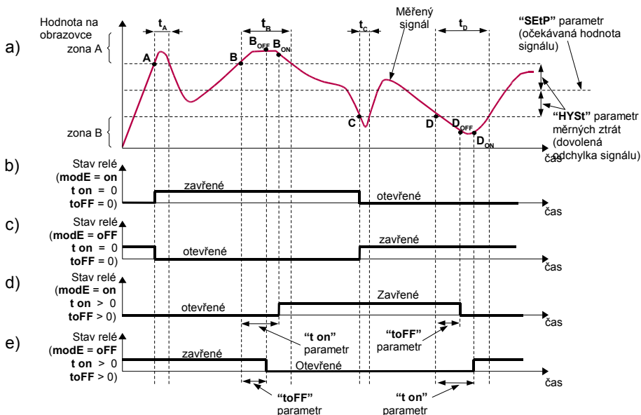
Obrázek 6.6. Zásady funkce výstupního relé (kontrolky LED)
