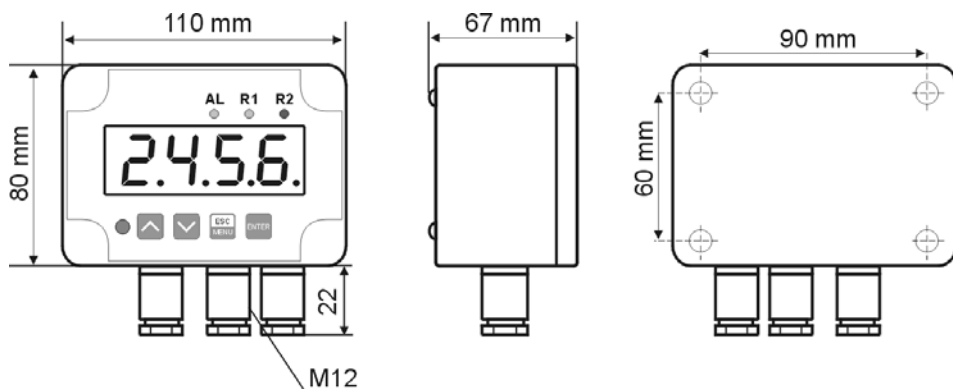
Obrázek 4.1. Rozměry jednotky
