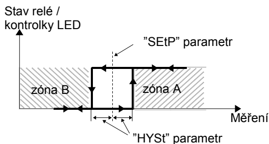
Obrázek 6.4. Jednoprahové řízení reléových výstupů a kontrolky LED R1÷R4
