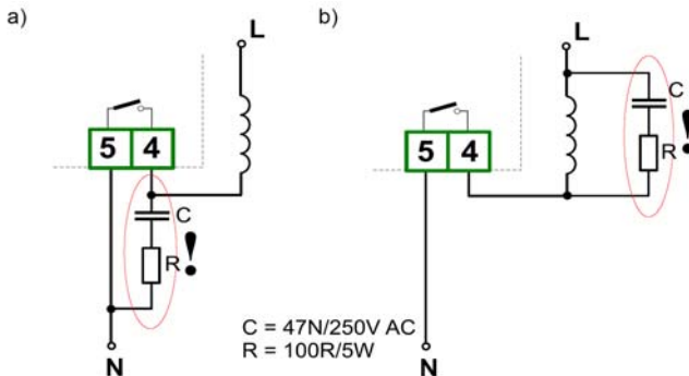
Obrázek 4.6. Příklady zapojení pro potlačení rušení vzniklého při rozpínání indukční zátěže a) RC členem na kontaktech relé b) RC členem na indukční zátěži
