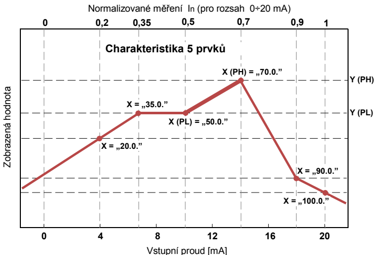
Obrázek. 8.4 Příklad charakteristiky definované uživatelem
