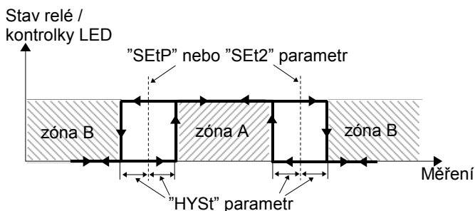
Obrázek 6.5. Dvouprahové řízení reléových výstupů a kontrolky LED R1÷R4
