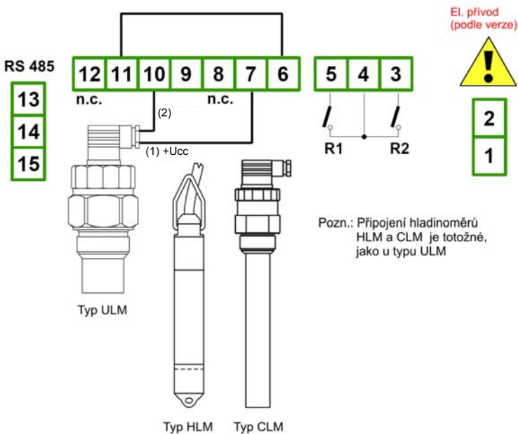
Obrázek 4.5. Schéma připojení hladinoměru k jednotce PDU
