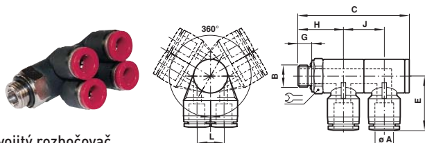
Dvojitý rozbočovač
