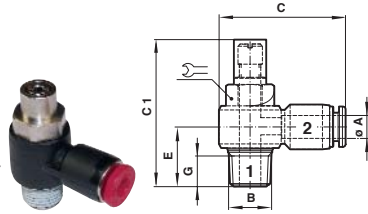
Otočné L-šroubení s regulací průtoku na výstupu
