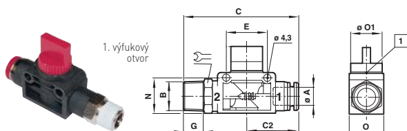
3/2 Uzavírací ventil
