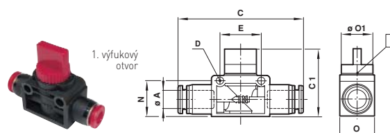
3/2 Uzavírací ventil
