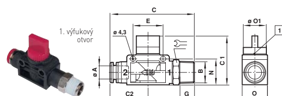
3/2 Uzavírací ventil
