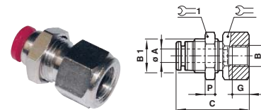
Přepážková přímá spojka (s vnitřním závitem)
