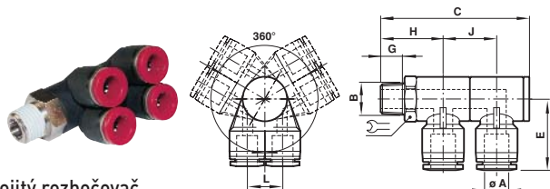
Dvojitý rozbočovač
