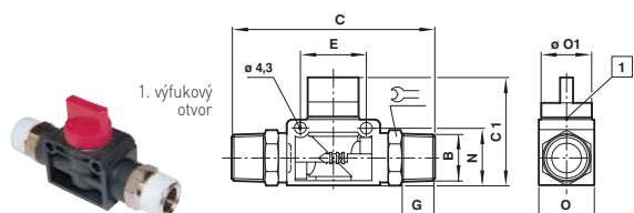
3/2 Uzavírací ventil
