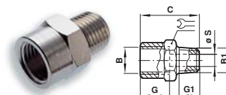
Redukční šroubení (s vnitřním a vnějším závitem) - redukce
