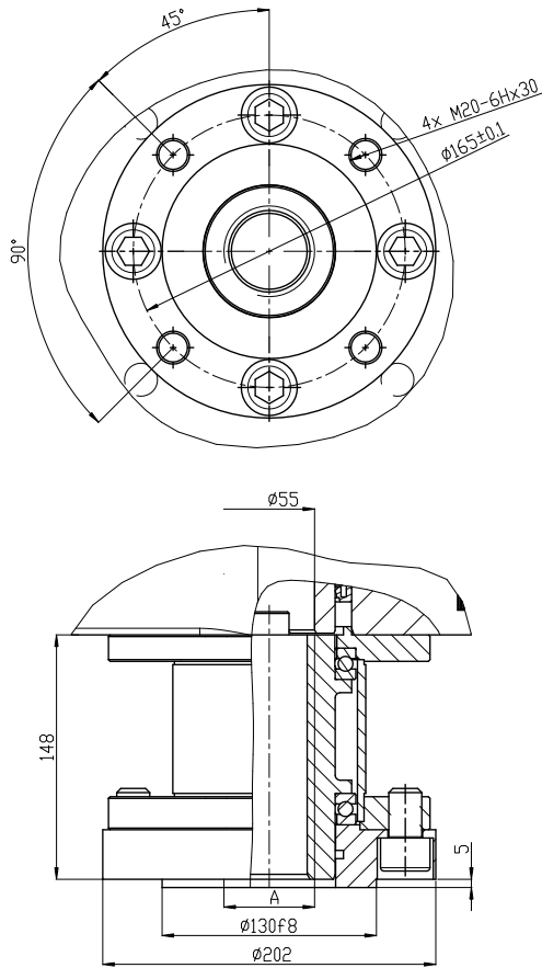
Rozmery adaptéra A / Adapter A - dimensions \
